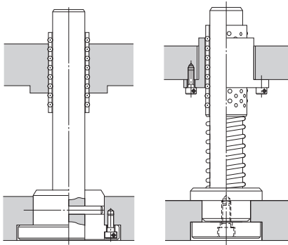
图2 安装例
