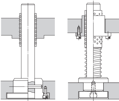
图2 安装例
