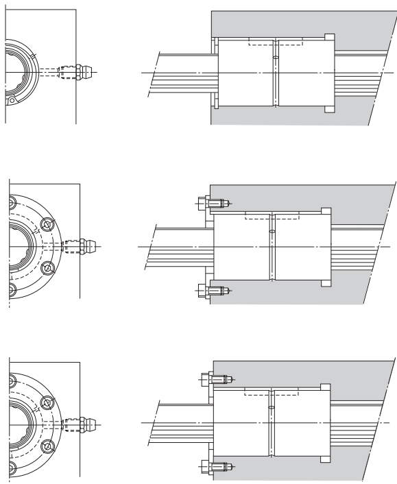
图1 花键母的安装例
