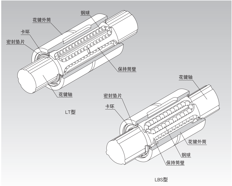
图1 滚珠花键LBS、LT型的结构
