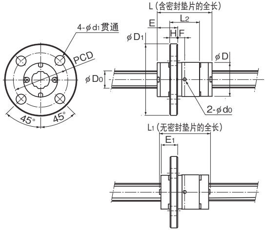
LF5X · LF5XL · LF6X · LF6XL · LF8X · LF8XL
