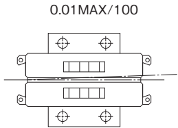
(c)LM滚柱滚动块和滚动面之间在水平方向的平行度
