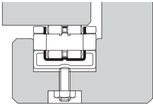
(a)使用专用弹性衬垫
