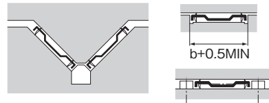
图5 引导板式滚柱链
