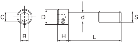
图3 专用安装螺栓
